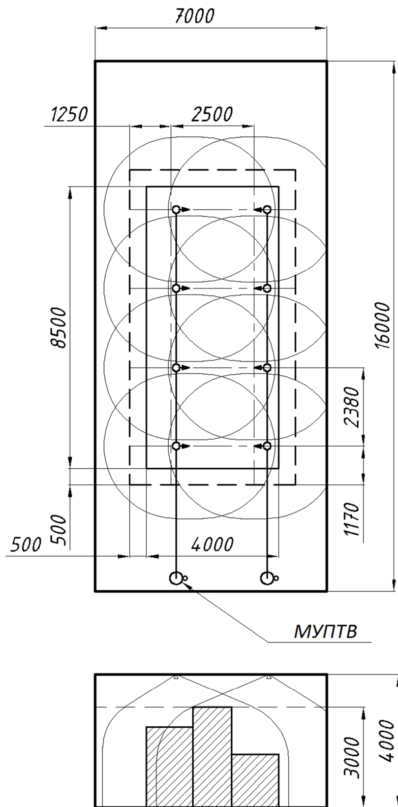
Рис. Г.9. Вариант размещения МУПТВ-160-Г-ВД с насадками-распылителями «НС-390-С» на плане защищаемого помещения.
