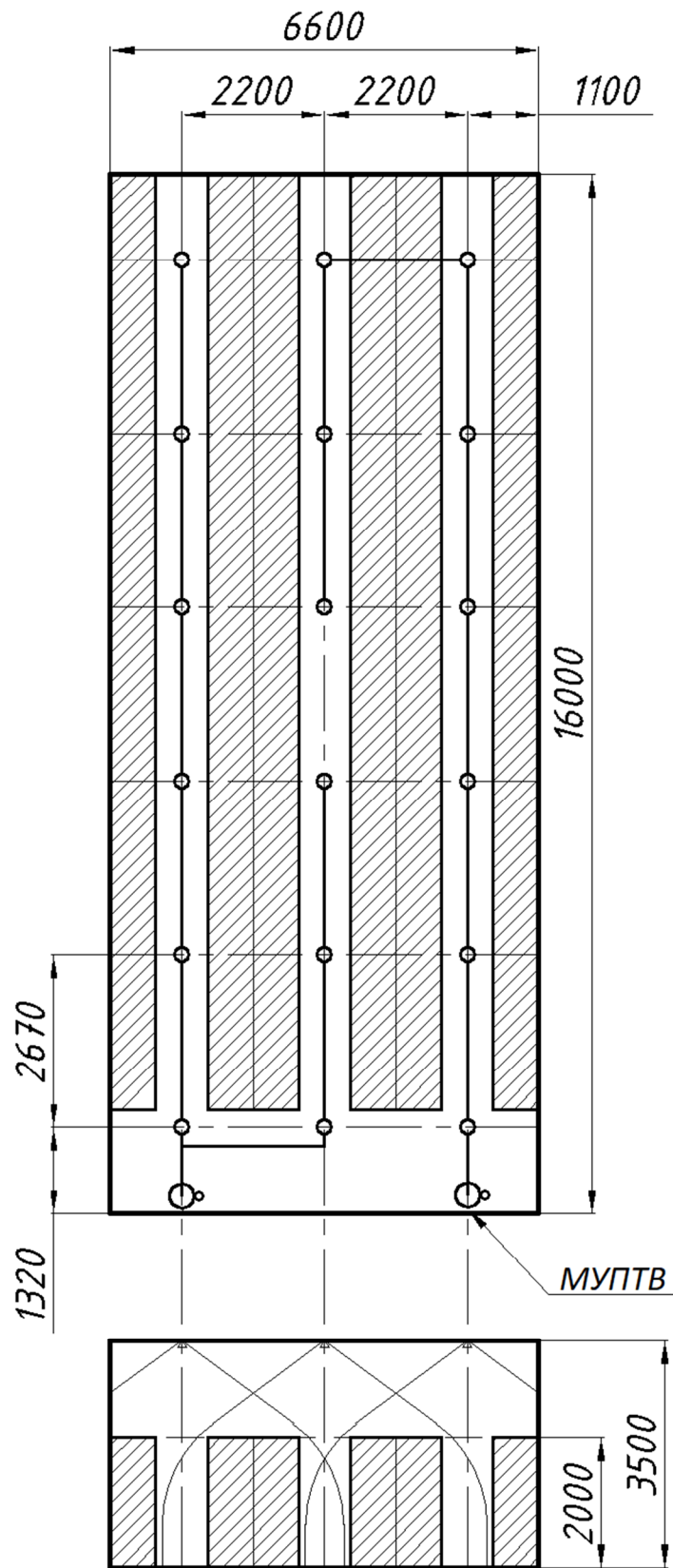
Рис. Г.10. Вариант размещения МУПТВ-160-Г-ВД с насадками-распылителями «НС-145» на плане защищаемого помещения.
