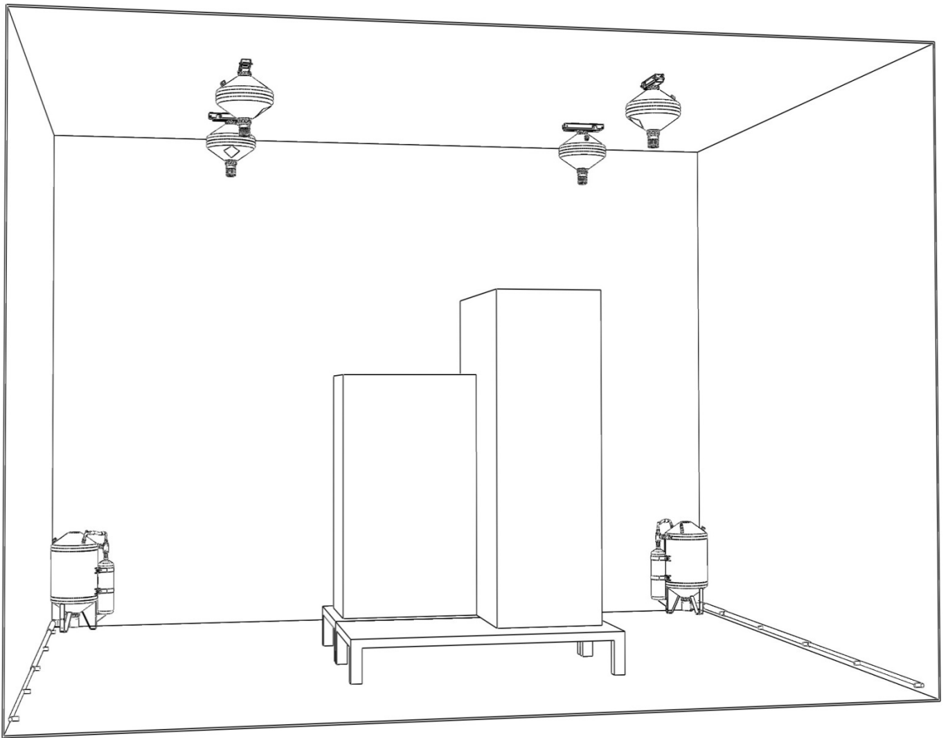
Рис. Ж.14. Вариант защиты помещения складского назначения с затененными зонами с применением МУПТВ-14,5-ГЗ-ВД и МУПТВ-50-Г-ВД.
