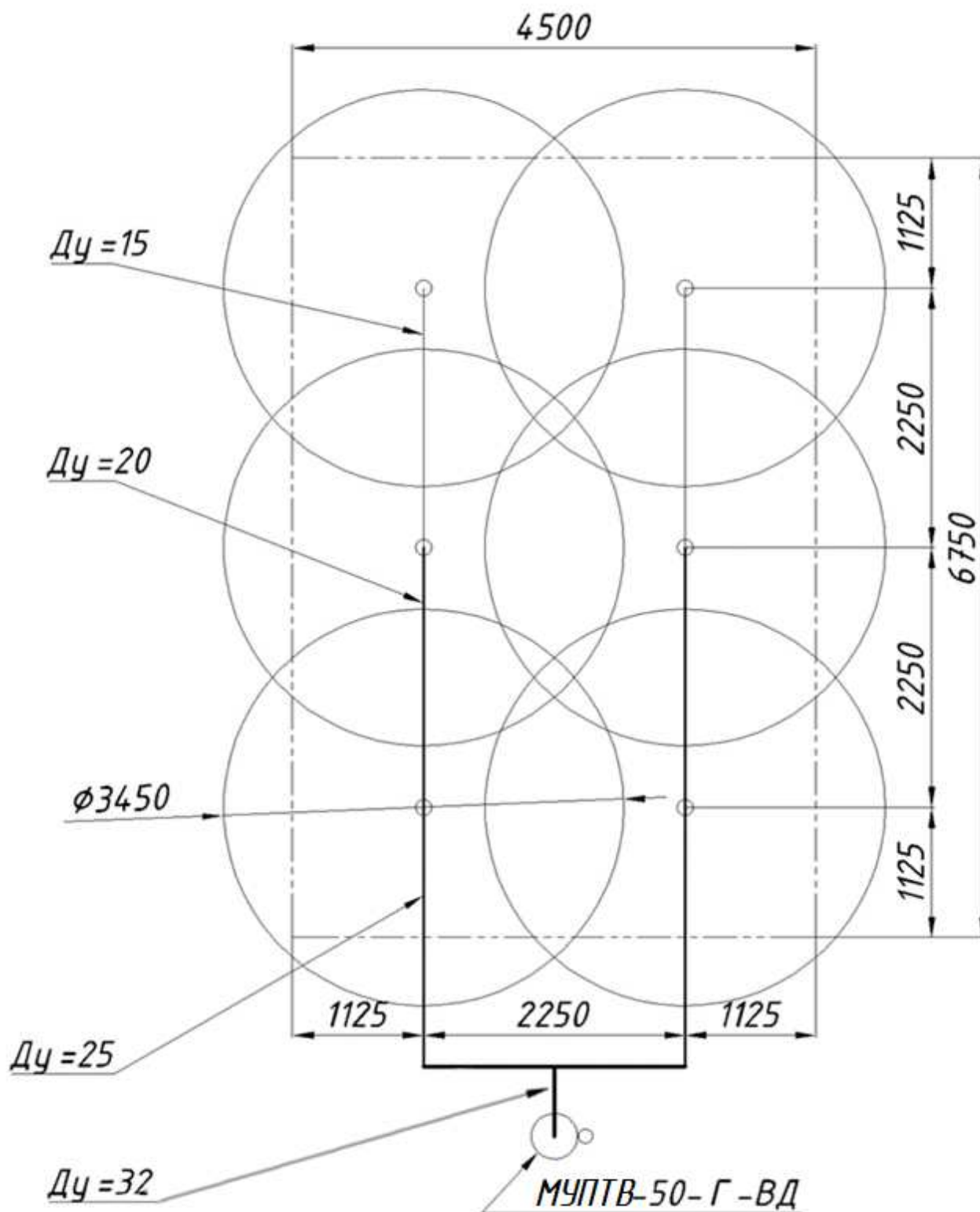
Рис. В.3. Пример зоны защиты одной МУПТВ-50-Г-ВД.
