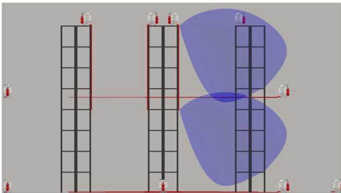
Рис. Ж.13. Вариант защиты помещения складского назначения с затененными зонами с применением МУПТВ-50-Г-ВД.
