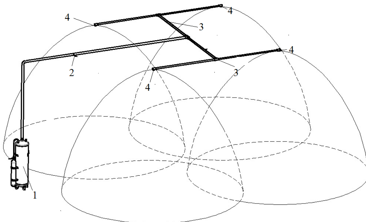
Рис.7.1 Принципиальная схема технологической части МУПТВ-160-Г-ВД или МУПТВ-50-Г-ВД.
