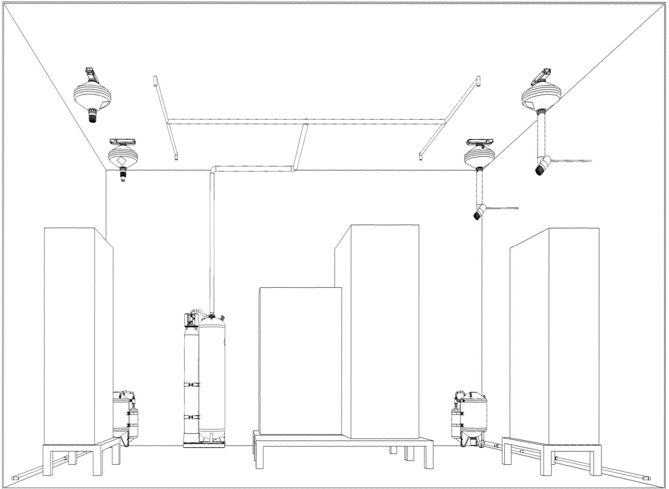
Рис. Ж.15. Пример защиты помещения складского назначения с затененными зонами с применением МУПТВ-14,5-ГЗ-ВД, МУПТВ-50-Г-ВД и МУПТВ-160-Г-ВД.
