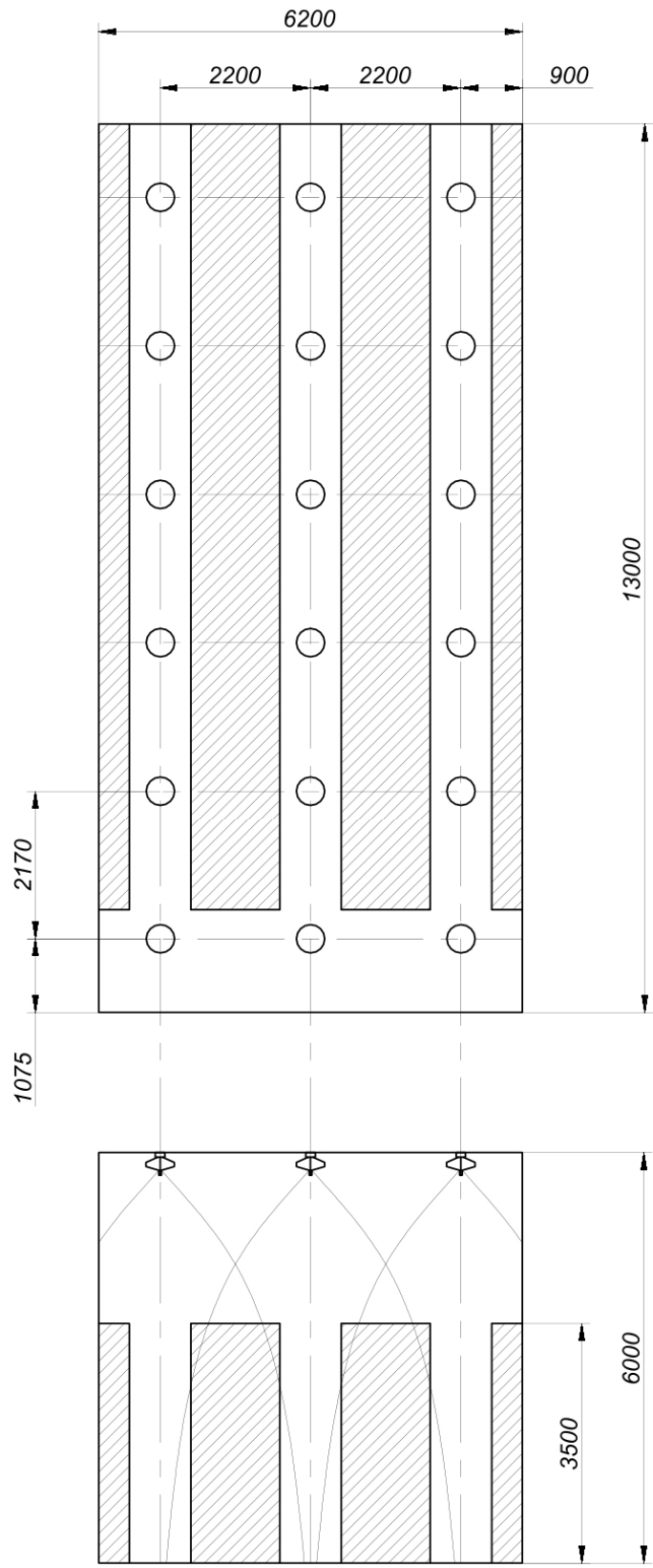
Рис. Б.13. План размещения МУПТВ в защищаемом помещении.
