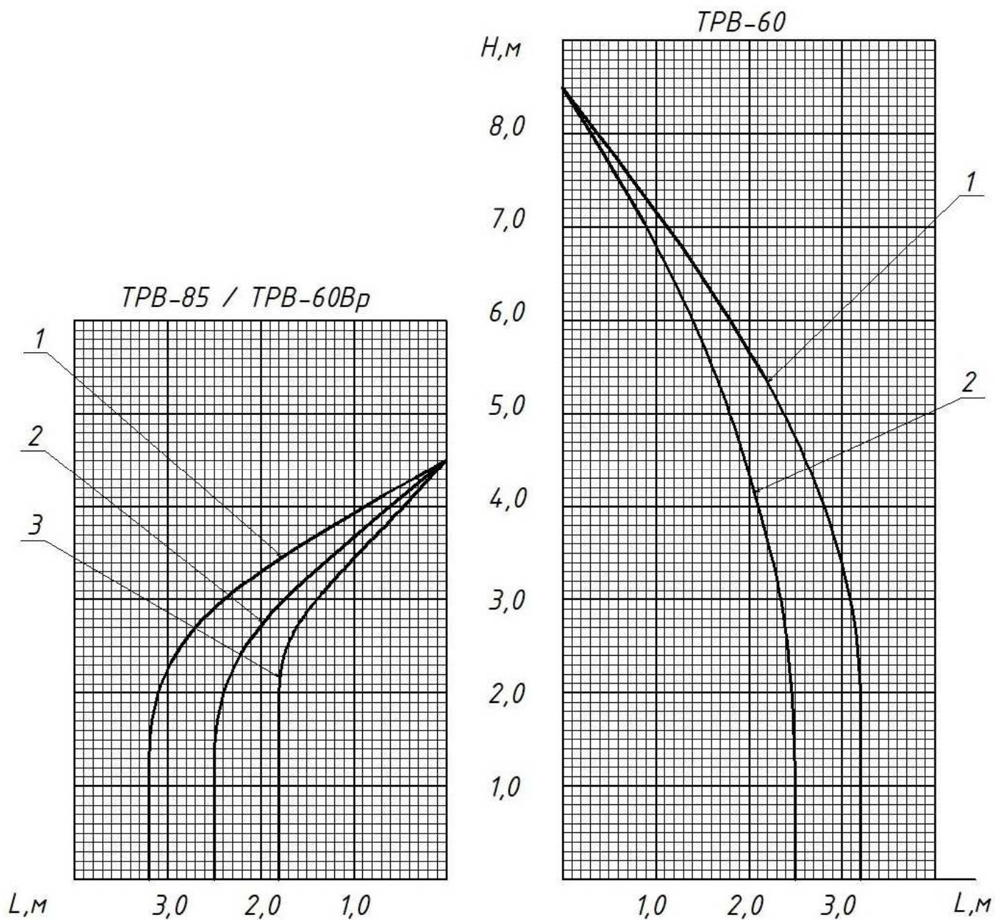
Рис. Б.2. Графики для определения радиуса орошения одиночного МУПТВ-14,5-ГЗ-ВД или МУПТВ-14,5-Г-В.
