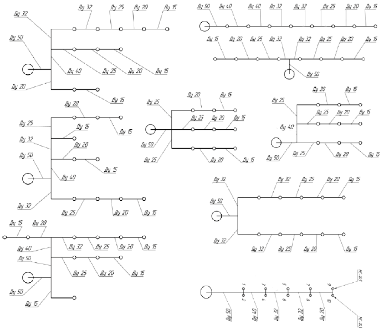
Рис. Г.3.2. Примеры схем проектирования трубопровода в составе МУПТВ-160-Г-ВД с насадками-распылителями «НС-145».
