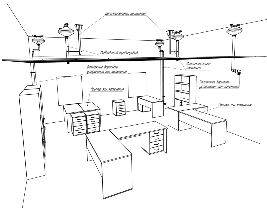
Рис.Ж.9. Вариант защиты помещения офисного назначения с затененными зонами с применением МУПТВ-14,5-ГЗ-ВД.
