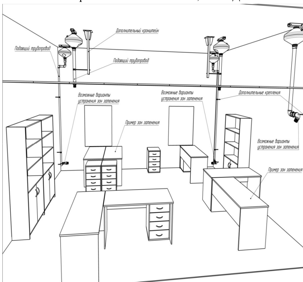
Рис.Ж.11. Вариант защиты помещения офисного назначения с затененными зонами с применением МУПТВ-14,5-ГЗ-ВД.
