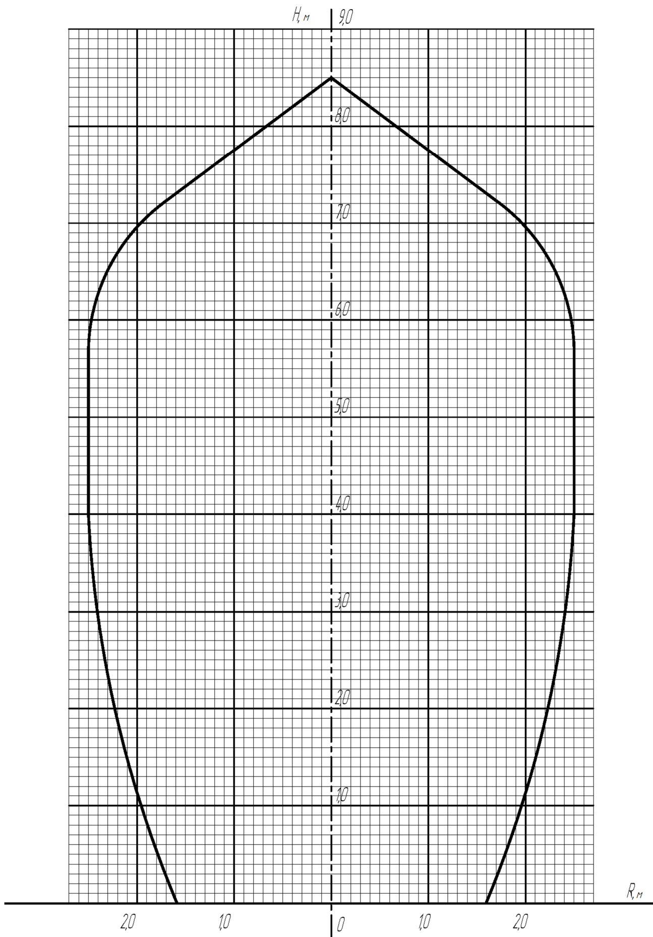
Рис. Г.1. Диаграмма орошения насадка-распылителя «НС-145» в составе МУПТВ-160-Г-ВД.
