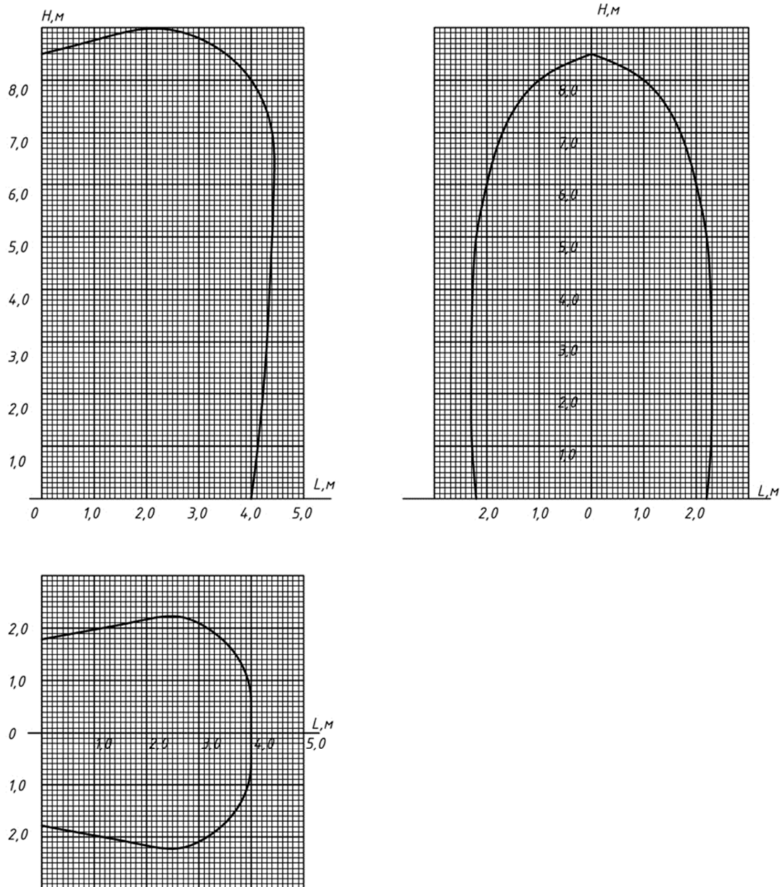
Рис.Г.7. Диаграмма орошения насадка-распылителя «НС-390-С» в составе МУПТВ-160-Г-ВД, расположенного под углом 45^\circ к вертикали.
