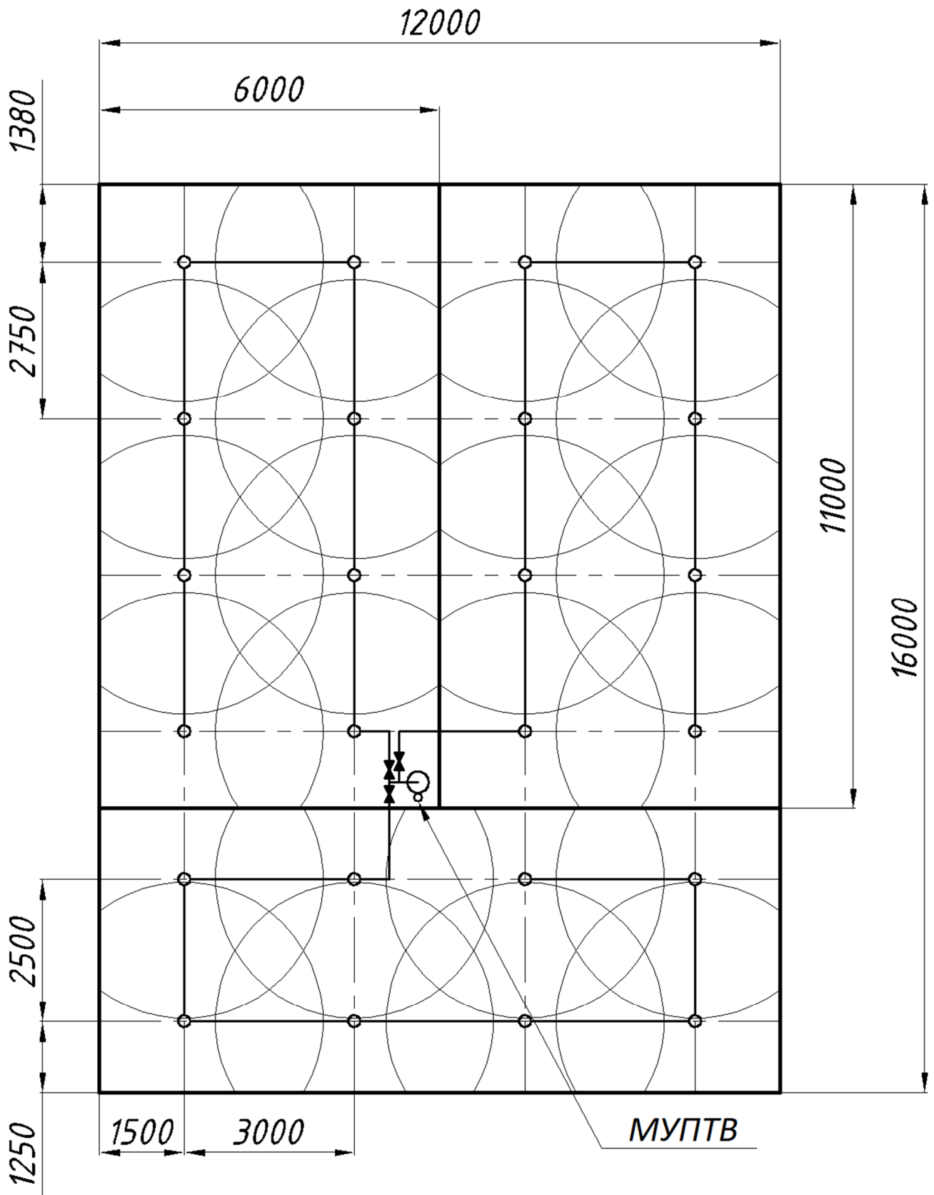
Рис.Г.12. Вариант размещения МУПТВ-160-Г-ВД по направлениям с насадками-распылителями «НС-145» на плане защищаемых помещений.
