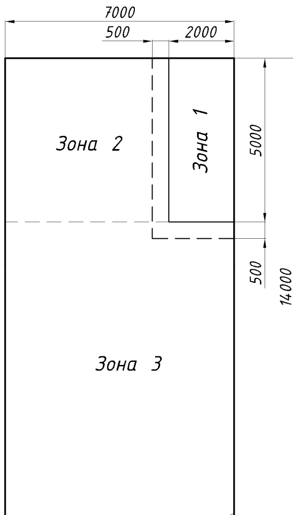
Рис. В.6. Разделение защищаемого помещения на зоны.
