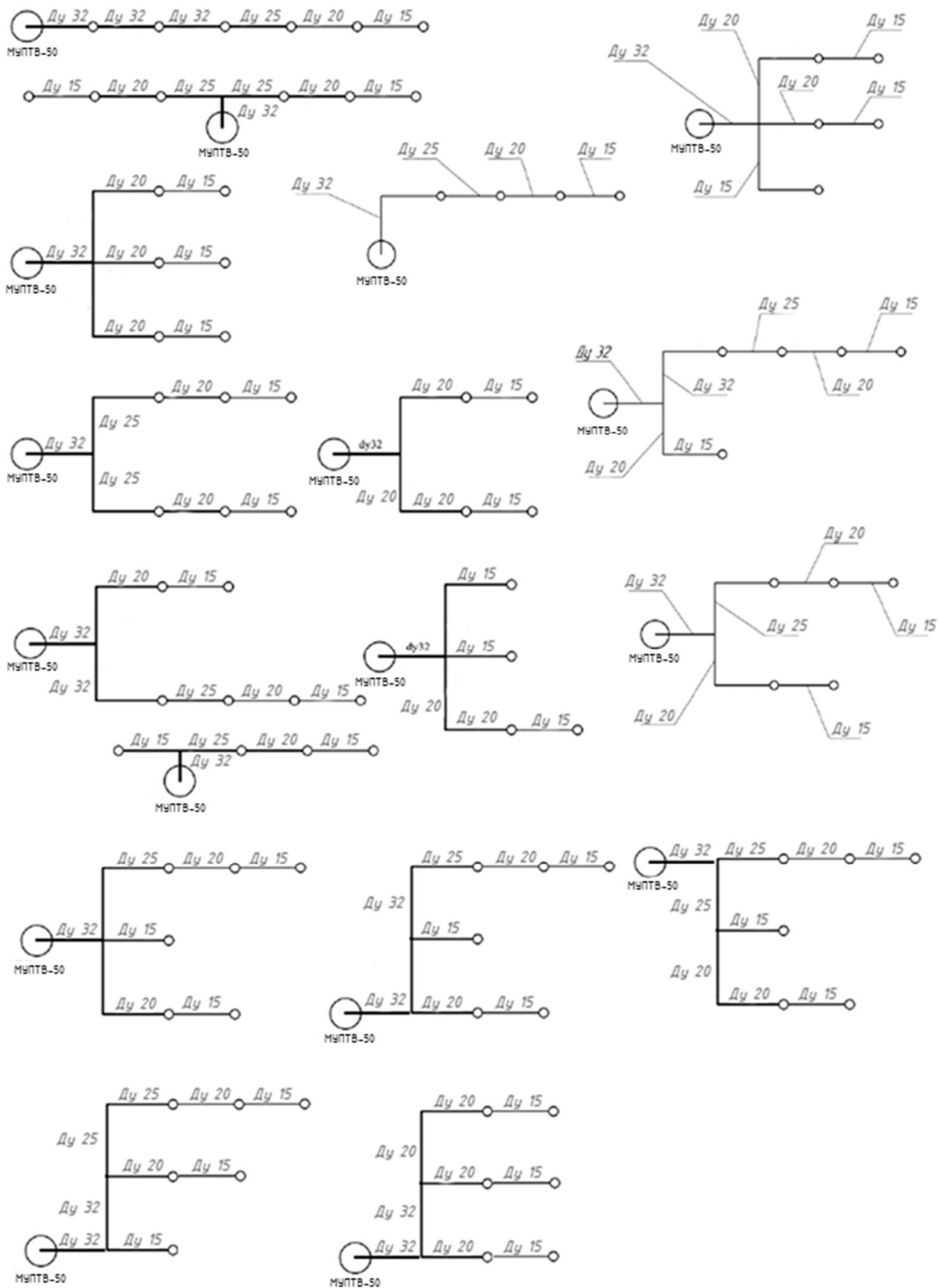
Рис. В.2. Рекомендуемые схемы проектирования трубопровода в составе МУПТВ-50-Г-ВД.
