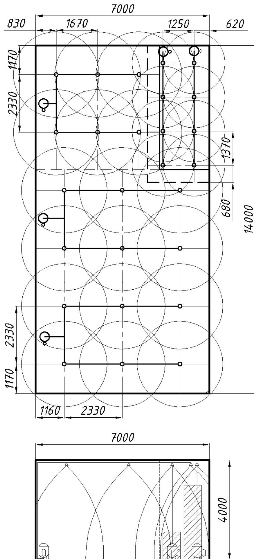
Рис.В.7. Вариант размещения МУПТВ-50-Г-ВД с насадками-распылителями «НС-145» на плане защищаемого помещения.
