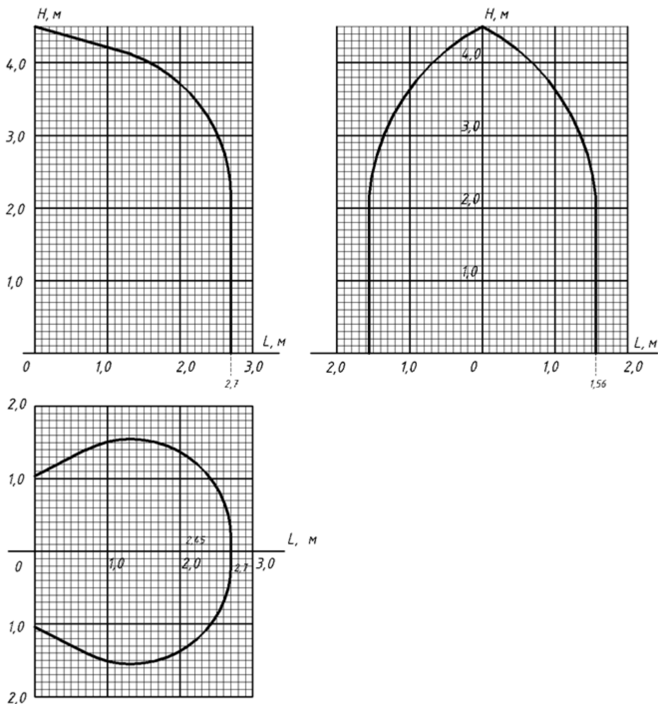
Рис.В.4. Диаграмма орошения насадка-распылителя «НС-145» в составе МУПТВ-50-Г-ВД, расположенного под углом 45^\circ к вертикали.
