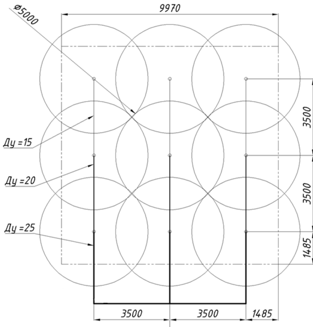
Рис. Г.4. Пример зоны защиты одной МУПТВ-160-Г-ВД с применением насадков-распылителей «НС-145».
