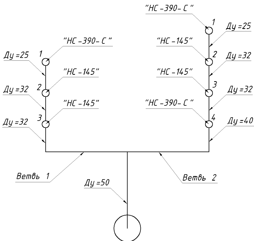
Рис.Д.1. Схема трубопровода МУПТВ-160-Г-ВД с применением различных типов насадков-распылителей.
