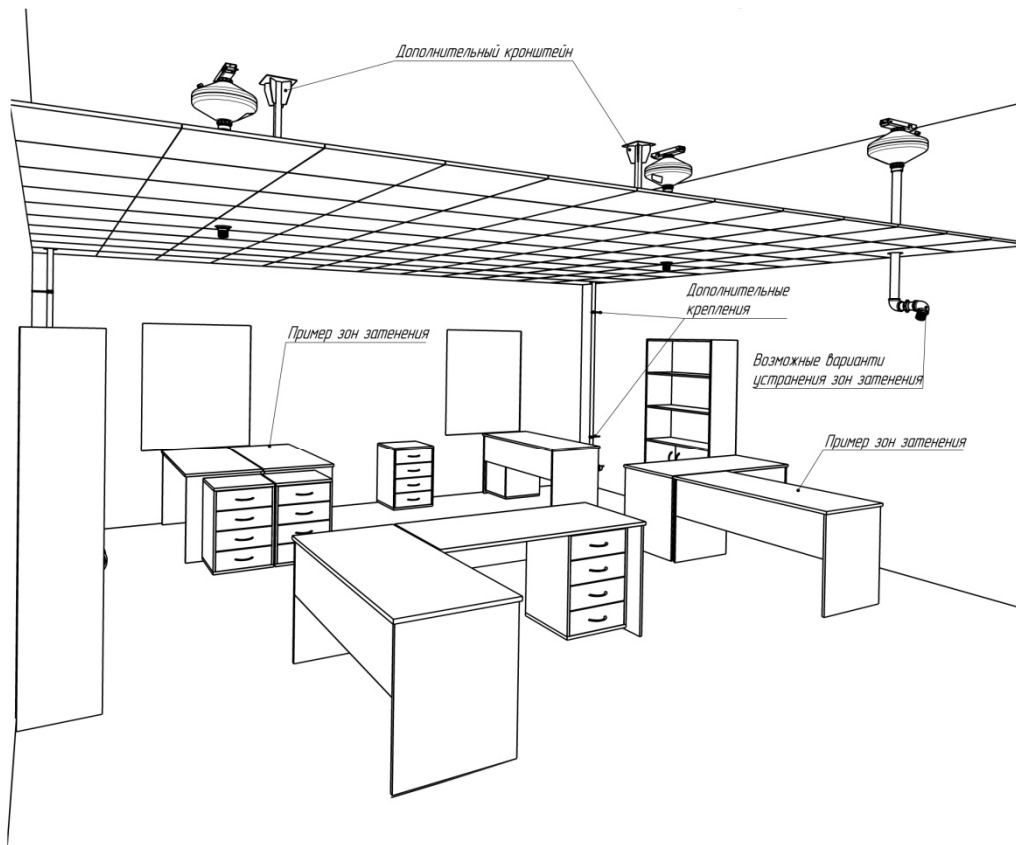
Рис.Ж.12. Вариант защиты помещения офисного назначения с затененными зонами с применением МУПТВ-14,5-ГЗ-ВД.
