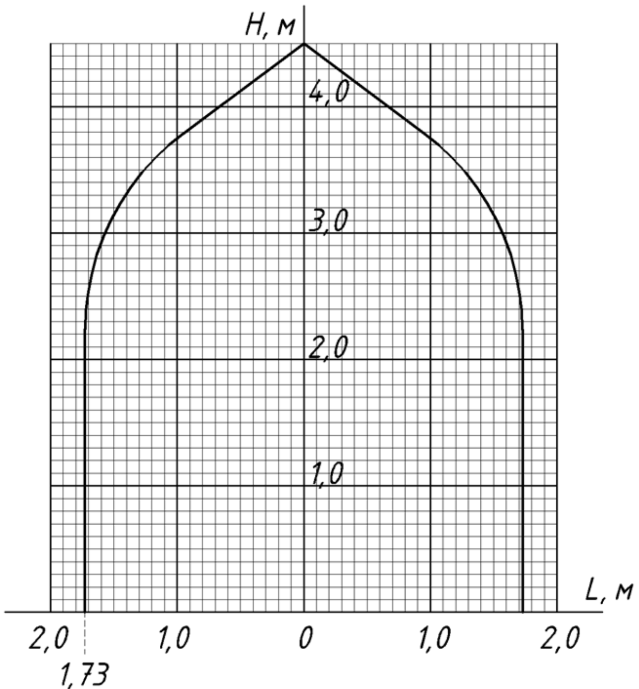
Рис. В.1. Диаграмма орошения насадка-распылителя «НС-145» в составе МУПТВ-50-Г-ВД.
