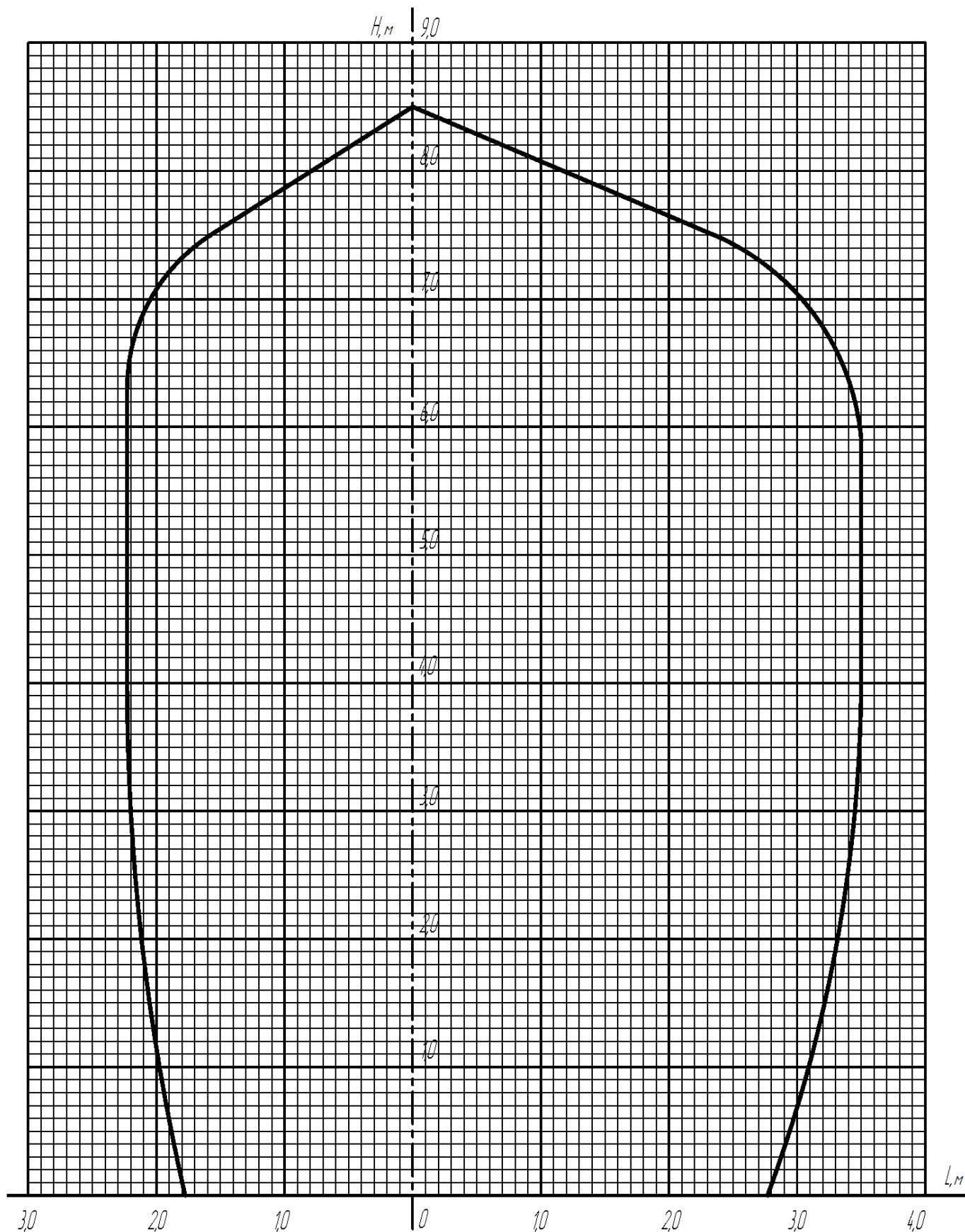
Рис. Г.2. Диаграмма орошения насадка-распылителя «НС-390-С» в составе МУПТВ-160-Г-ВД.
