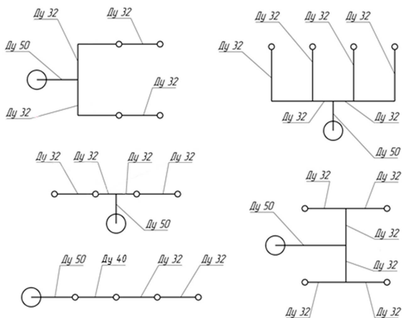
Рис. Г.3.1. Рекомендуемые схемы проектирования трубопровода в составе МУПТВ-160-Г-ВД с насадками-распылителями «НС-390-С».
