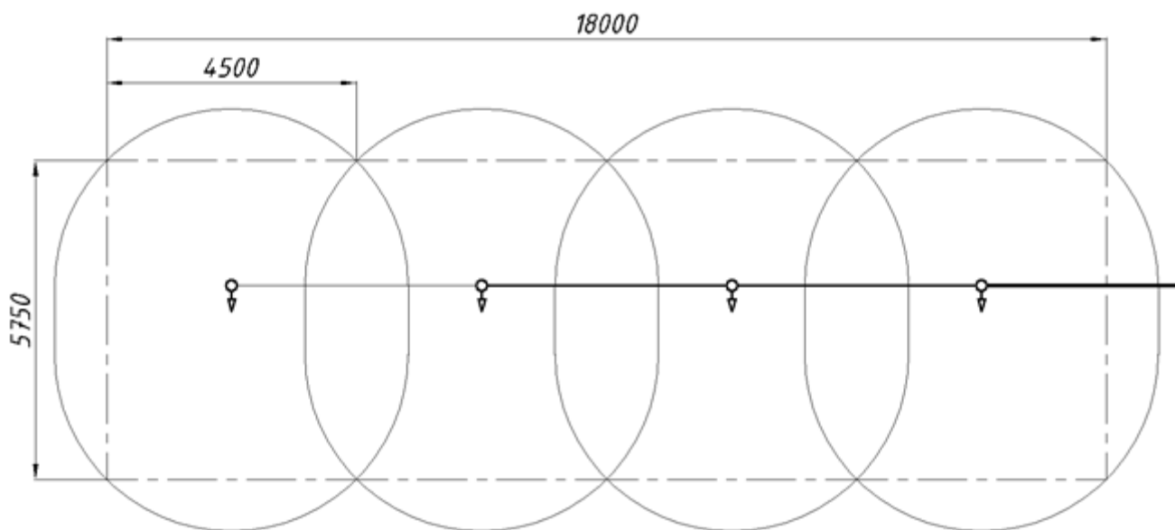
Рис. Г.5. Пример зоны защиты одной МУПТВ-160-Г-ВД с применением насадков-распылителей «НС-390-С».
