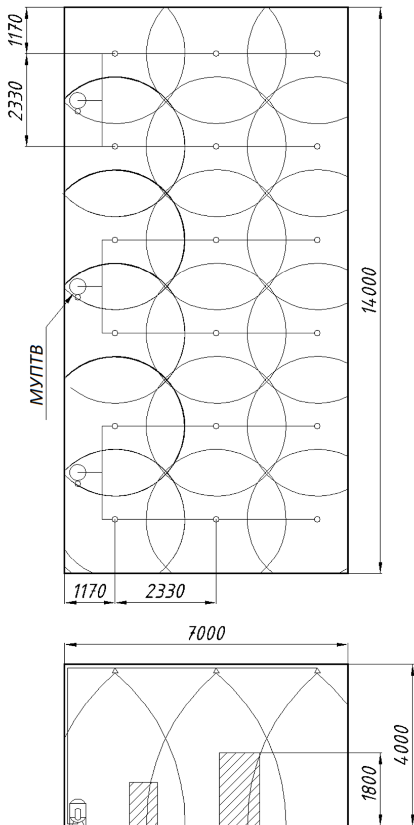
Рис.В.5. Вариант размещения МУПТВ-50-Г-ВД с насадками-распылителями «НС-145» на плане защищаемого помещения.
