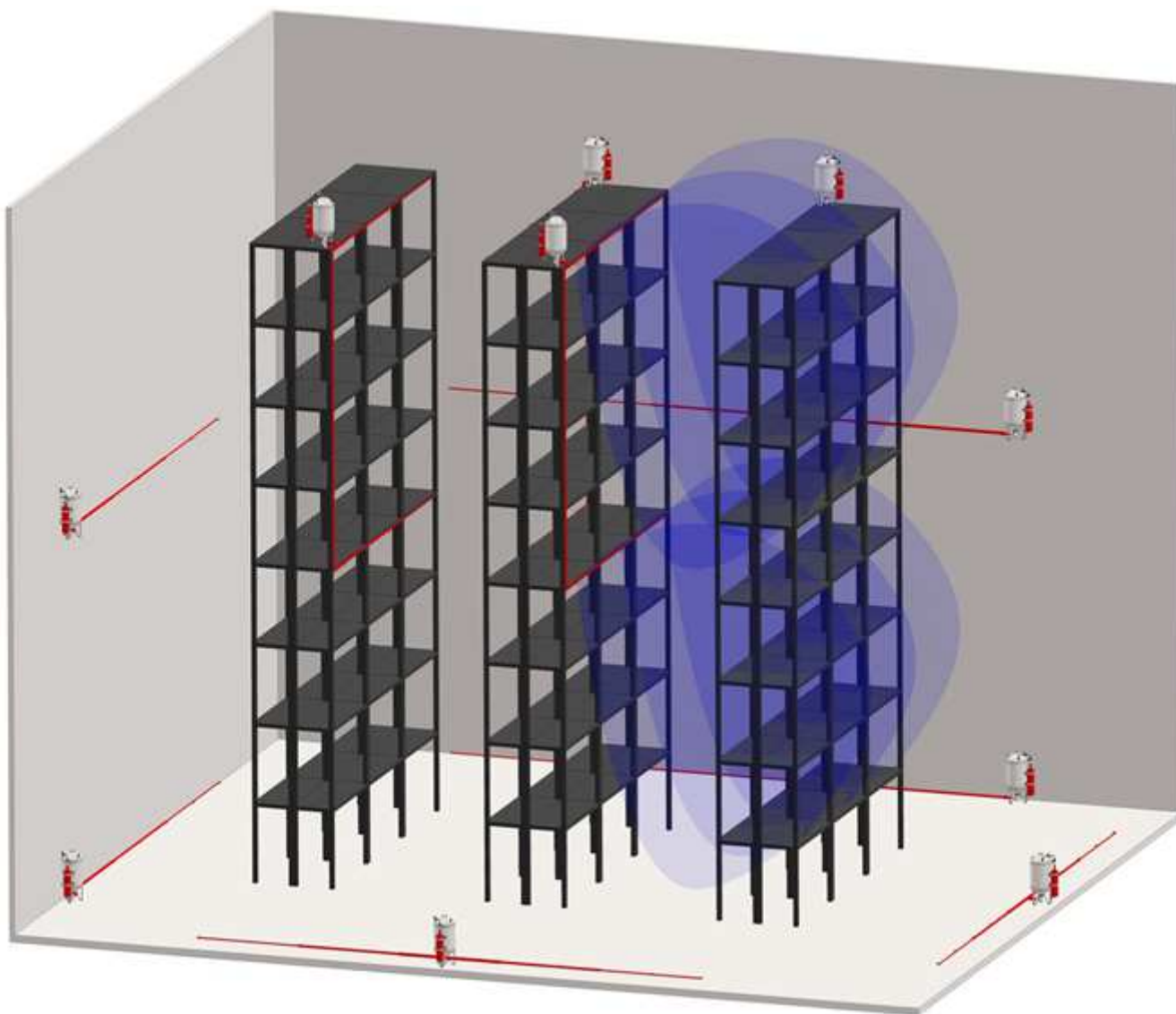
Рис. Ж.13. Вариант защиты помещения складского назначения с затененными зонами с применением МУПТВ-50-Г-ВД.
