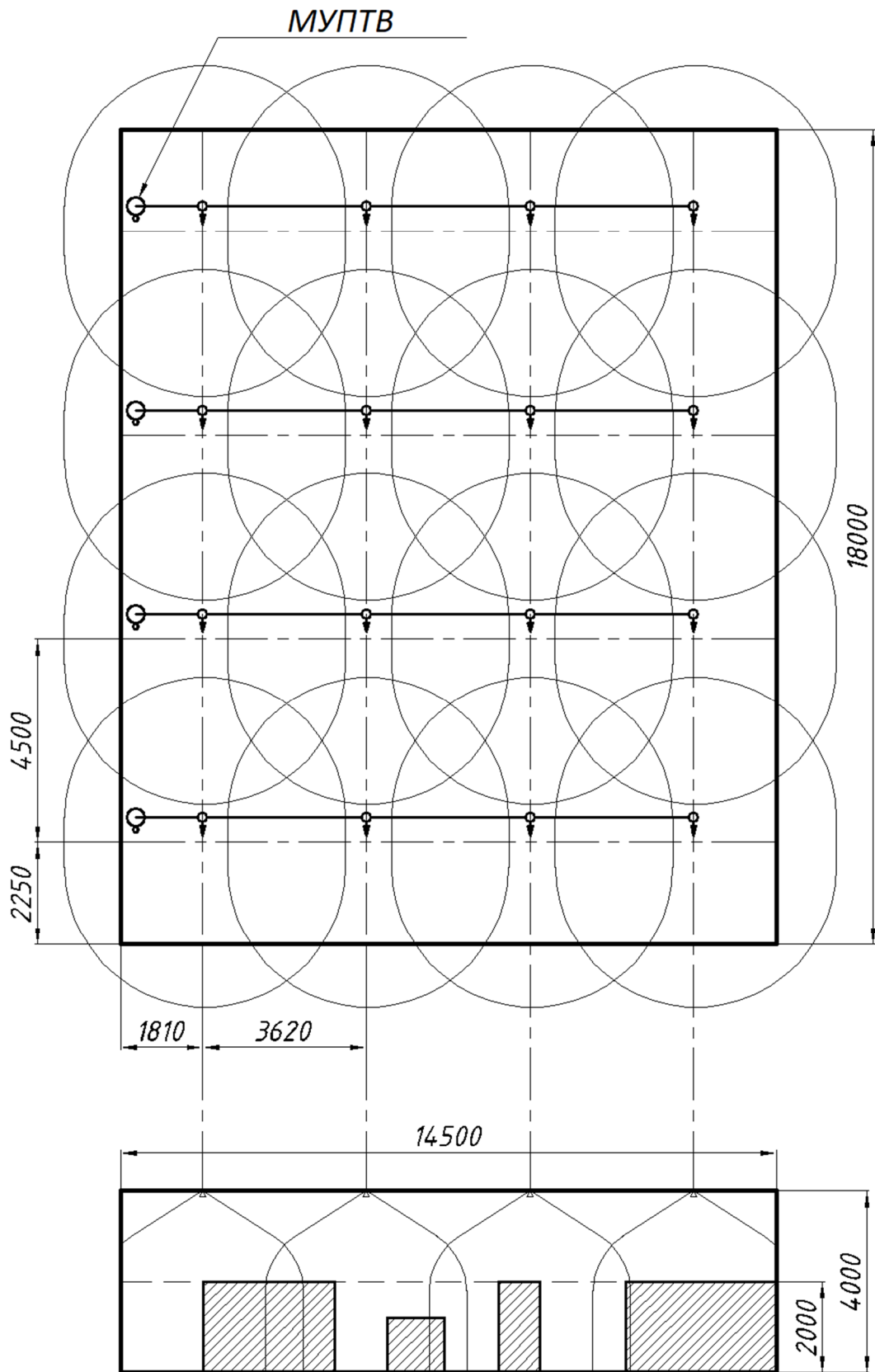
Рис. Г.8. Вариант размещения МУПТВ-160-Г-ВД с насадками-распылителями «НС-390-С» на плане защищаемого помещения.
