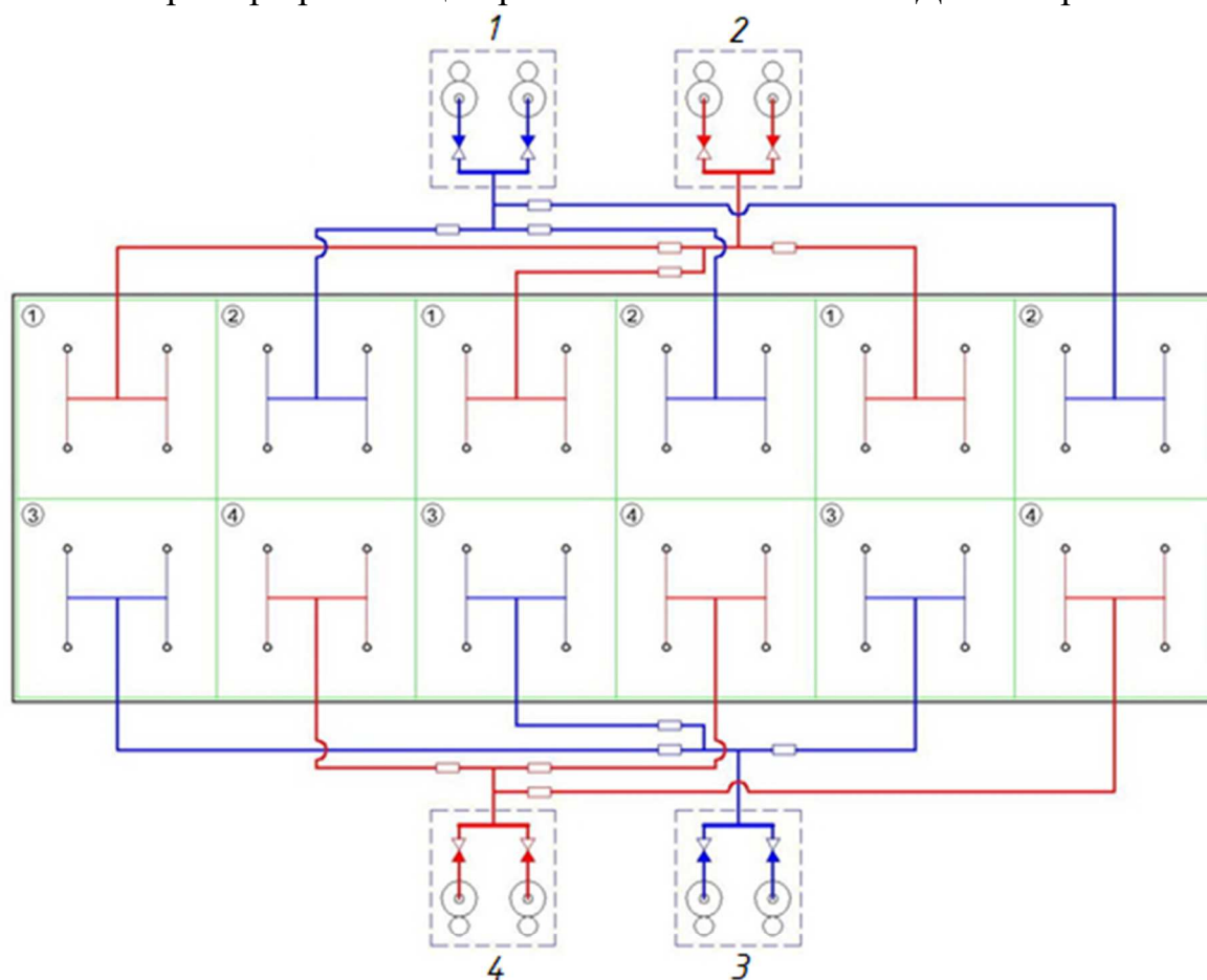
Рис. 7.3. Пример организации работы МУПТВ-160-Г-ВД по направлениям.
