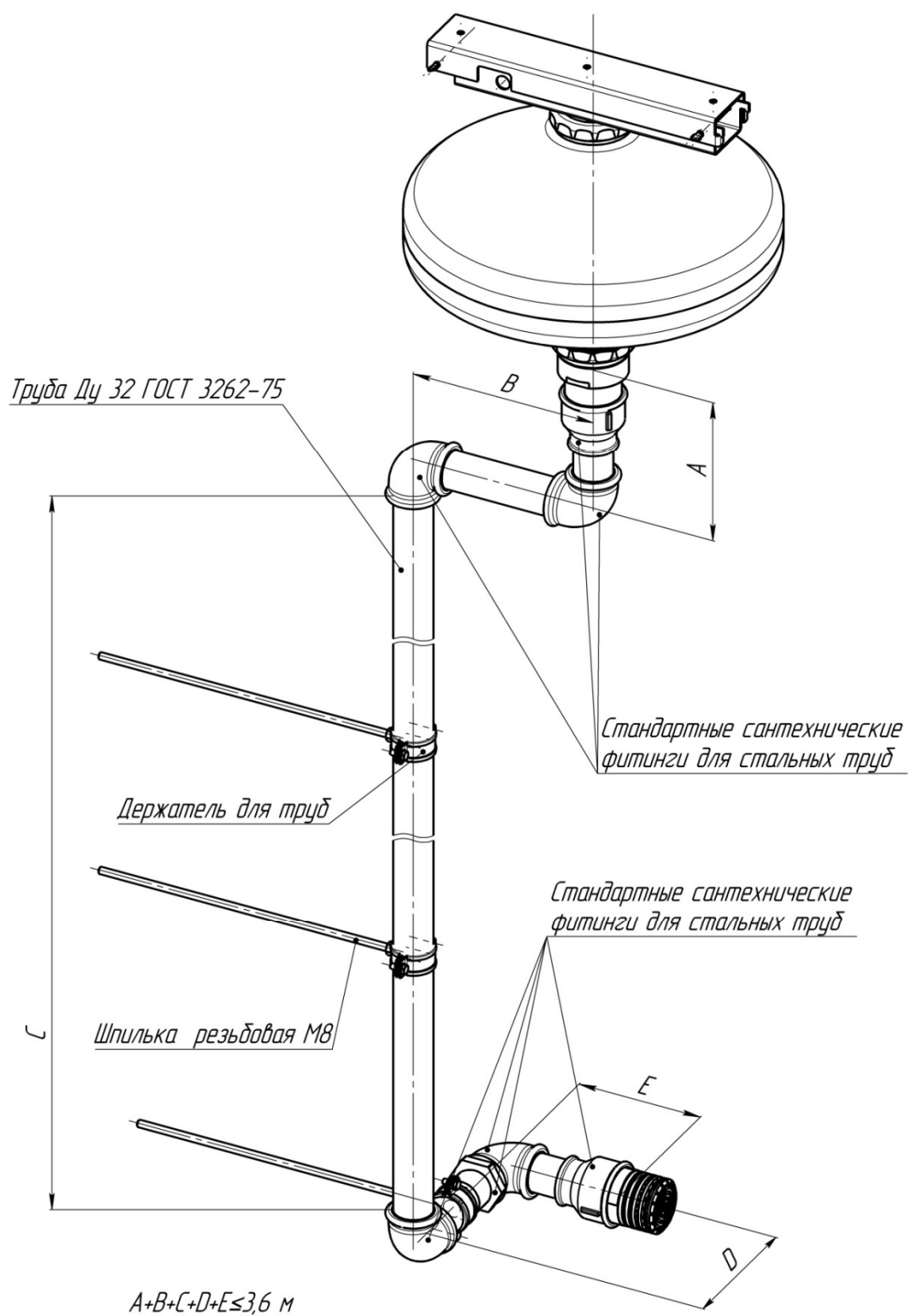
Рис.Ж.3. Пример использования удлинительного трубопровода с диаметром проходного сечения 32 мм в составе МУПТВ-14,5-ГЗ-ВД.
